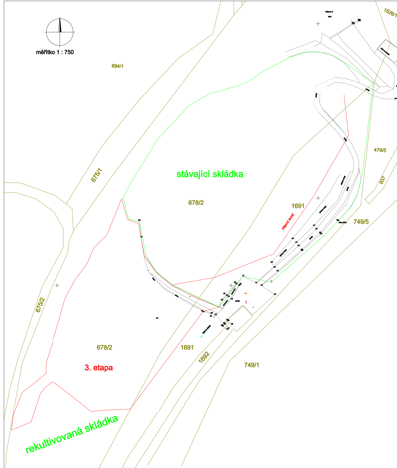
Rozšíření skládky Č. Krumlov - 3. etapa
