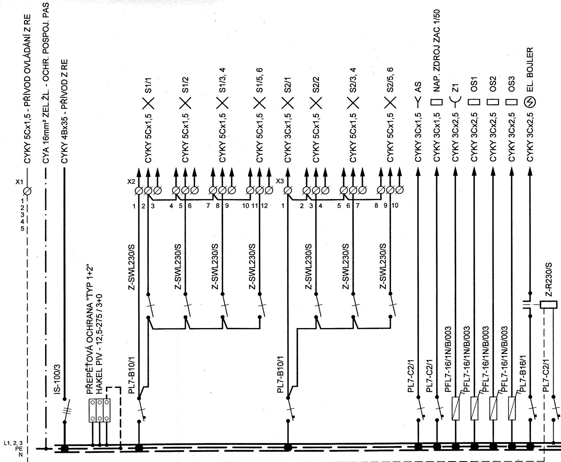
RT - L1, 2, 3 + PE + N; 3x 230/400V; 50Hz
