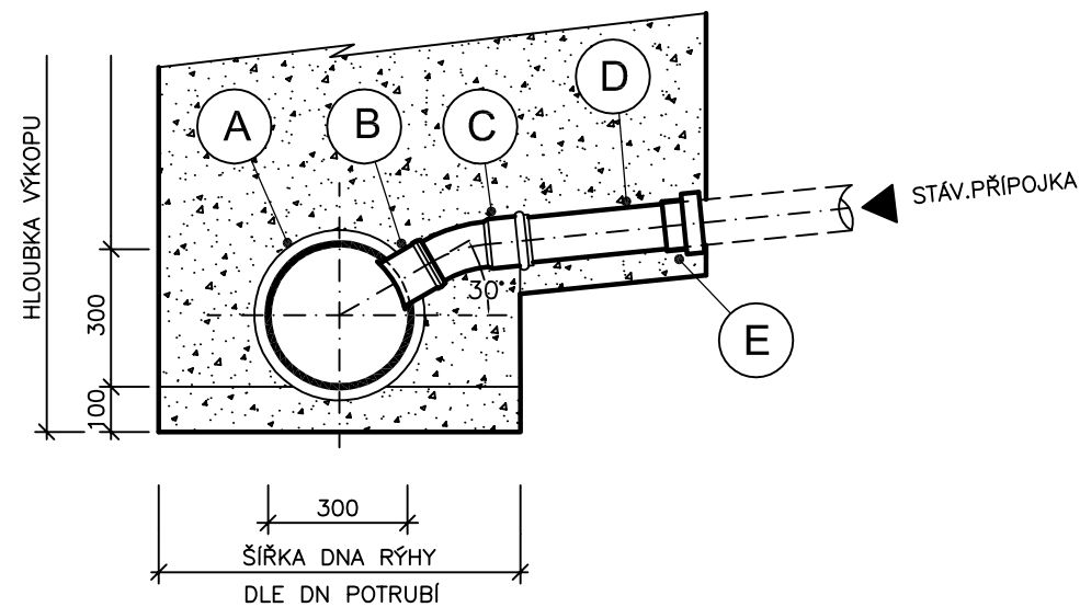
PŘÍČNÝ ŘEZ
