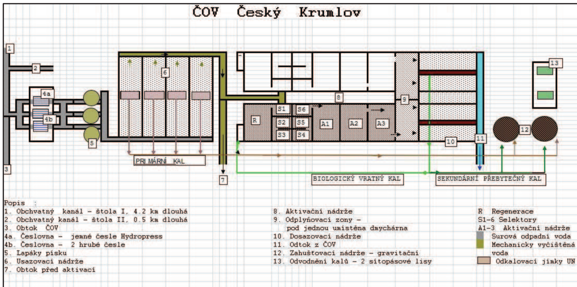
Příloha č. 2 – Schéma ČOV
