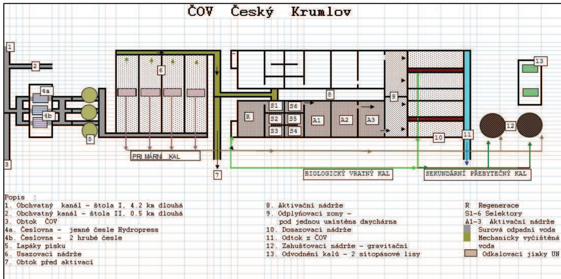
Příloha č. 1 – Schéma ČOV
